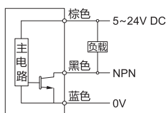
接线图
