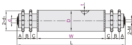
平端面型 QCH26/27
