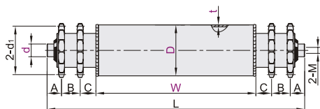
标准型 QCH28/29
