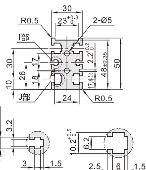
I部放大图(M3用) J部放大图(M6用)
