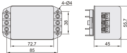
导轨安装 ZHN55
