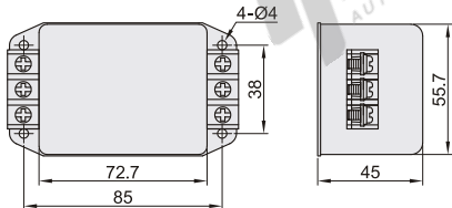
螺丝固定 ZHN54
