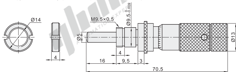
Y-HCA02 (行程: 0~13)(最小读数: 0.01) (带安装螺母)
