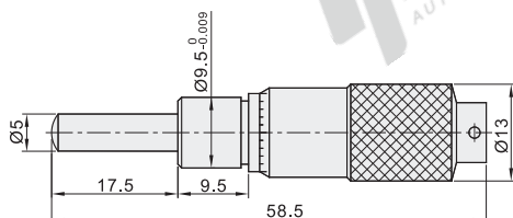
Y-HCA21 (行程: 0~13)(最小读数: 0.01)
