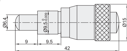
Y-HCA14 (行程: 0~6.5)(最小读数: 0.005)
