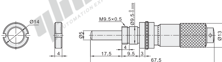
Y-HCA24 (行程: 0~13)(最小读数: 0.01) (带安装螺母)
