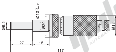
Y-HCA33 (行程: 0~25)(最小读数: 0.01)
