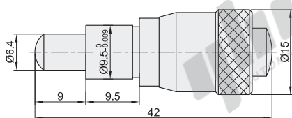
Y-HCA13 (行程: 0~6.5)(最小读数: 0.01)
