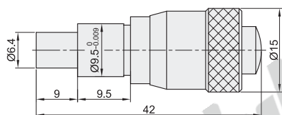
Y-HCA15 (行程: 0~6.5)(最小读数: 0.01)
