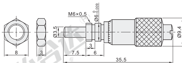
Y-HCA12 (行程: 0~6.5)(最小读数: 0.01) (带安装螺母)
