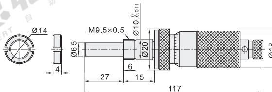
Y-HCA34 (行程: 0~25)(最小读数: 0.01) (带安装螺母)
