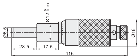
Y-HCA33 (行程: 0~25)(最小读数: 0.01)
