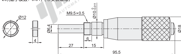
Y-HCA36 (行程: 0~25)(最小读数: 0.01) (带安装螺母)
