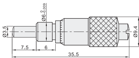
Y-HCA11 (行程: 0~6.5)(最小读数: 0.01)
