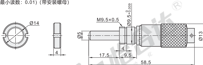
Y-HCA23 (行程: 0~13)(最小读数: 0.01) (带安装螺母)
