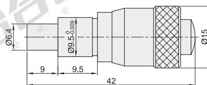
Y-HCA16 (行程: 0~6.5)(最小读数: 0.005)
