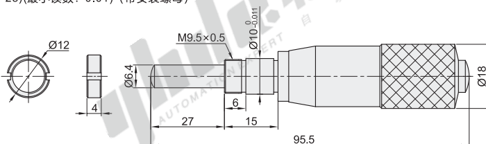
Y-HCA38 (行程: 0~25)(最小读数: 0.01) (带安装螺母)
