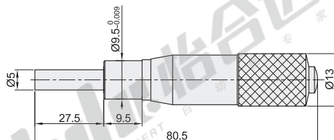
Y-HCA35 (行程: 0~25)(最小读数: 0.01)
