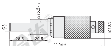
Y-HCA34 (行程: 0~25)(最小读数: 0.01) (带安装螺母)
