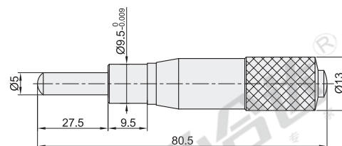
Y-HCA37 (行程: 0~25)(最小读数: 0.01)
