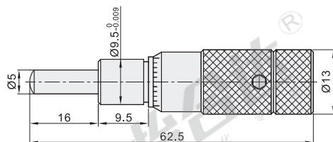
Y-HCA01 (行程: 0~13)(最小读数: 0.01)
