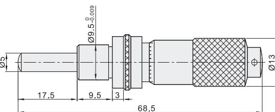
Y-HCA22 (行程: 0~13)(最小读数: 0.01)
