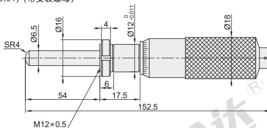
Y-HCA41 (行程: 0~50)(最小读数: 0.01) (带安装螺母)
