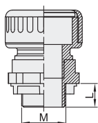
直接头
