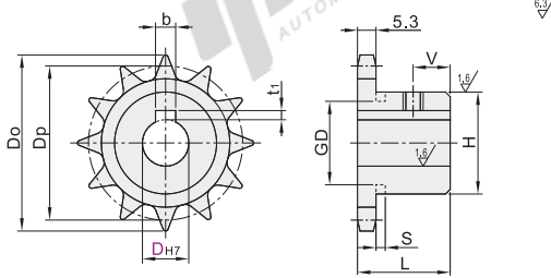
链轮 VLY01/02
