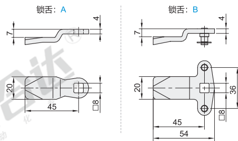
XAT23、XAT24锁舌形状
