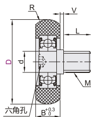
内六角外螺纹型 BKR62
