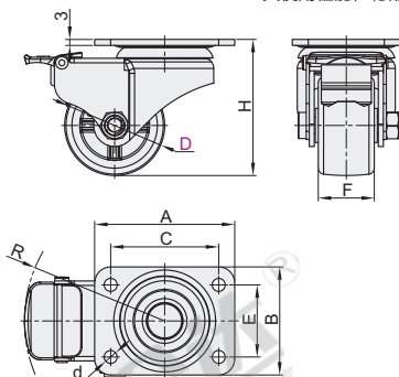
五金单刹 J-CRB03
