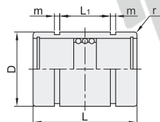
单衬型 Y-GVK01
