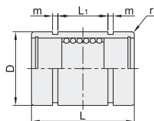
双衬型 Y-GVK11
