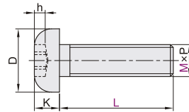
梅花槽盘头螺钉 TAU33/34/35
