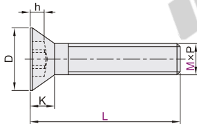
梅花槽沉头螺钉 TAU30/31/32
