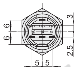
插脚位置图
