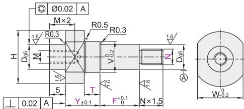
带挡圈槽型
