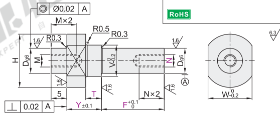
两端内螺纹型 Y-KCC84
