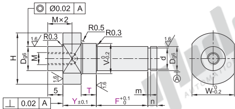
一端内螺纹一端外螺纹型 Y-KCC86
