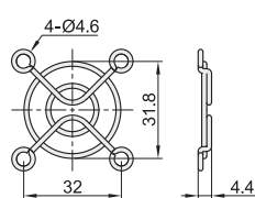
防护网 ZHJ42/45
