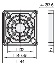
过滤网 ZHJ41
