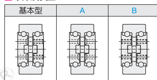
安装孔类型
