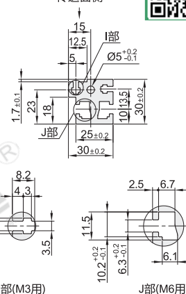
型材截面放大图 传送面侧
