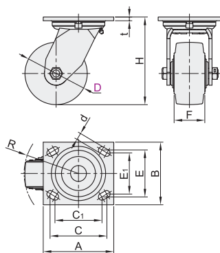
无刹 CEL02
