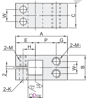
螺纹垂直型
