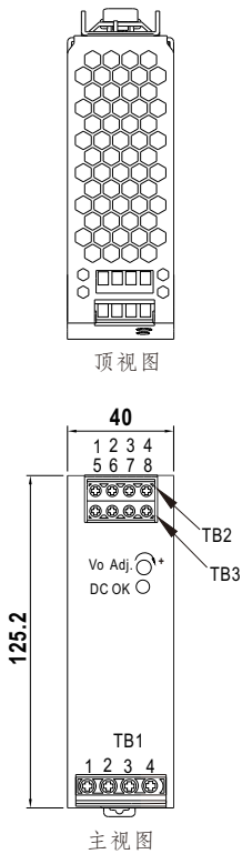
主视图
