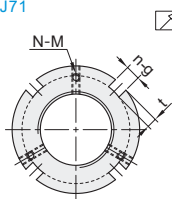
轴向锁紧型 BKJ71
