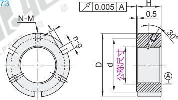
牙腹锁紧型 BKJ73
