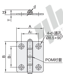
4孔安装
