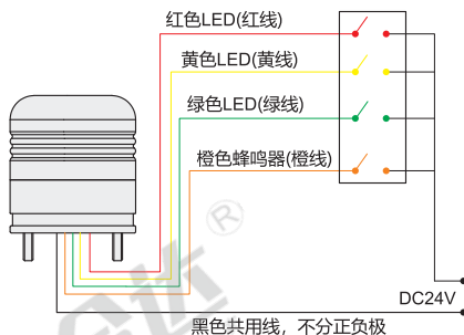
接线图
