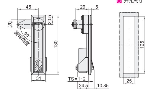
带锁芯 XAT71
