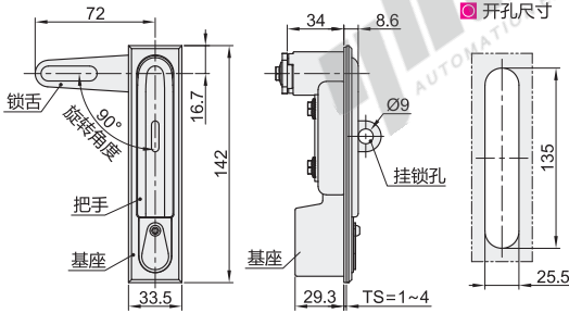
带锁芯带挂锁型 XAT59
