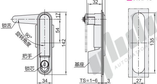
带锁芯 XAT72
