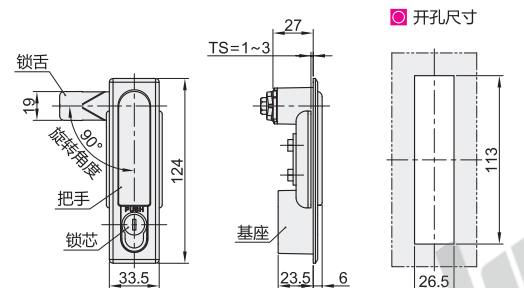
带锁芯 XBT67/68
