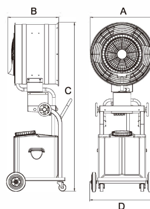
AMF-60 外形尺寸图
