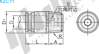
内六角孔直接头 XZC11
