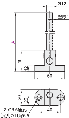
单管可调 ZLP70
