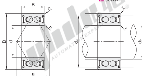
安装图
