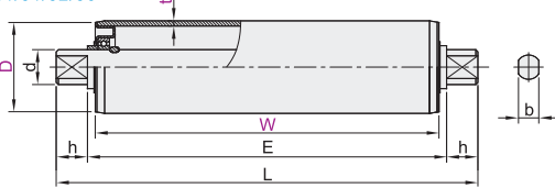
弹簧压入式-W尺寸选择型
