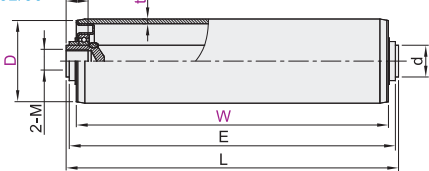
弹簧压入式-W尺寸指定型
