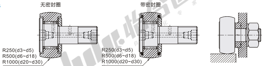
球面型 E-BPF25/26/35
