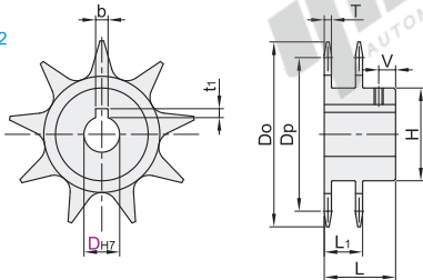
链轮 VLW02
