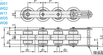
链条
