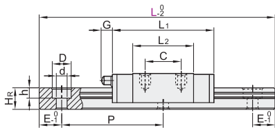
H(16) 带注油嘴
