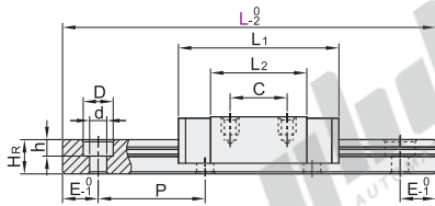
H(8 10 13) 带注油孔
