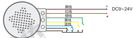
第一路触发(黄线) 第三路触发(蓝线) 第二路触发(绿线) 第四路触发(白线) 公共触发线(黑线)
