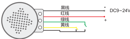
第一路触发(黄线) 第二路触发(绿线) 公共触发线(黑线)
