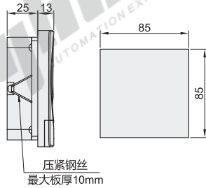
安装开孔尺寸
