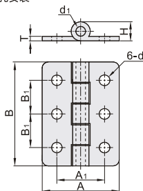
6孔安装
