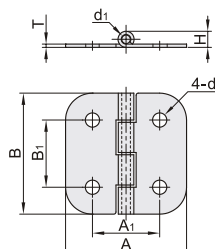
HFV16 4孔安装
