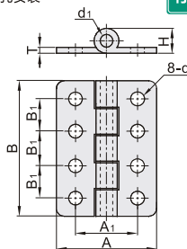
8孔安装
