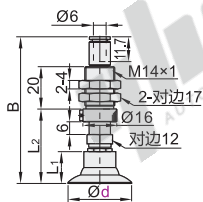
弹簧式顶部真空端口 J-WET66/67
