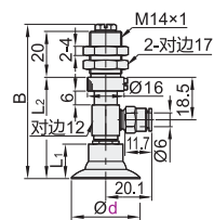
弹簧式侧面真空端口 J-WET71/72
