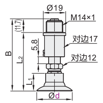
弹簧式直接安装型 J-WET76/77
