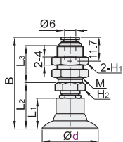
固定式顶部真空端口 J-WET61/62
