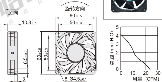
外形尺寸: 6010
