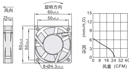
外形尺寸: 60/60B12
