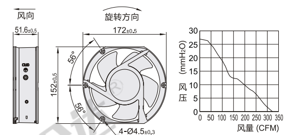
外形尺寸: 172
