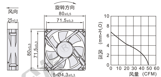
外形尺寸: 80/80B12/80B48
