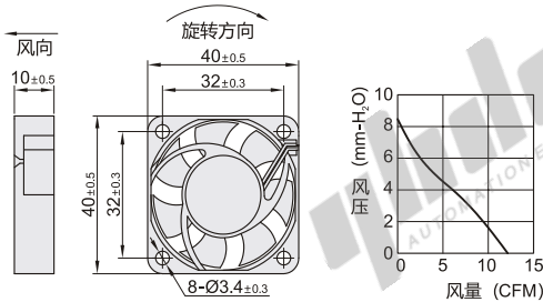
外形尺寸: 4010
