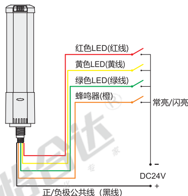
接线图
