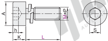
弹簧垫圈
