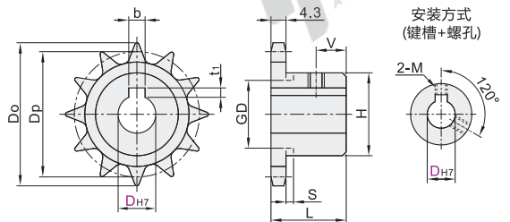
链轮 E-VLD02
