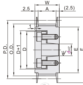
带轮形状 F形
