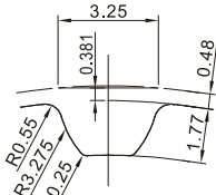
标准齿形
