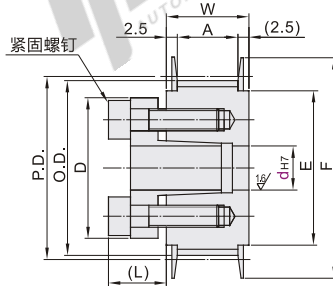
带轮形状 E形
