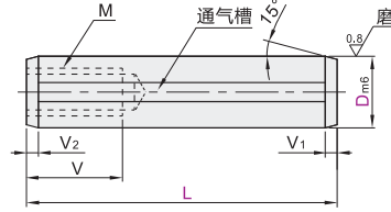
公差 m6 Y-KCF46-m6
