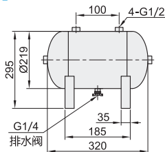
底架安装孔尺寸
