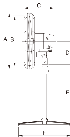
落地式外形尺寸图
