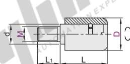
外螺纹型 HAB26
