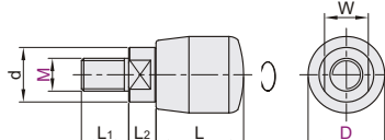
外螺纹带扳手槽型 HAB31
