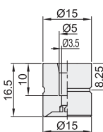
外径D: 15
