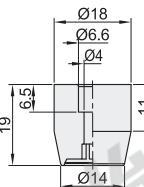
外径D: 18
