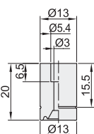
外径D: 13
