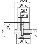
外径D: 16
