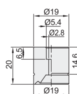
外径D: 19
