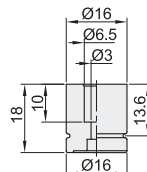
外径D: 16
