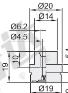
外径D: 19
