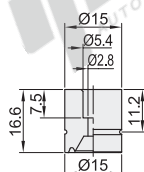
外径D: 15
