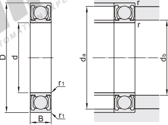
安装图
