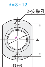
对边法兰型 Y-GVB21
