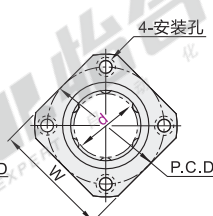
方法兰型 Y-GVB41
