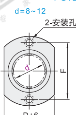
对边法兰型 Y-GVB51
