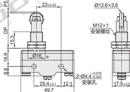
L(小竖轮柱塞型)
