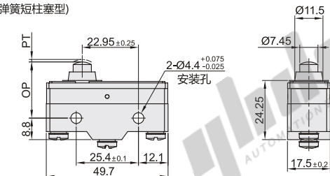
1(弹簧短柱塞型)
