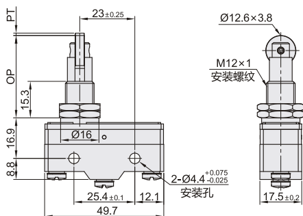
M(面板安装横向滚轮柱塞型)
