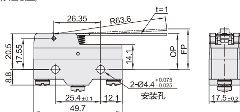
C(长压板型)
