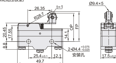
F(滚轮短压板型)
