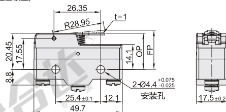
D(短压板型)
