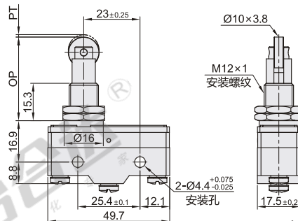
L(小竖轮柱塞型)
