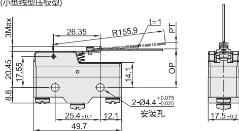
G(小型线型压板型)
