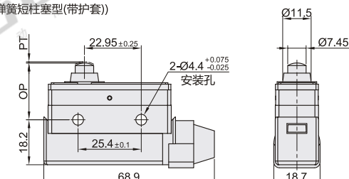
N(彈簧短柱塞型(帶护套))
