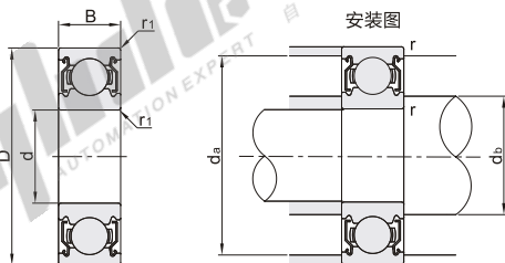
安装图
