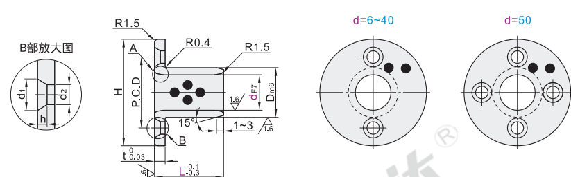
锥孔型 E-OF02
