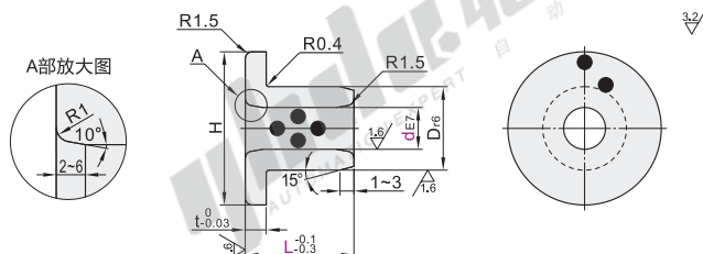
标准型 E-OF01
